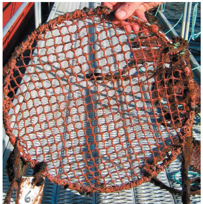
Prøving som er impregnert med Netwax NI Gold. Bildet er tatt etter at prøven har stått 8 måneder i sjøen.
